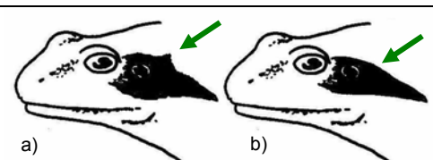
2.att. a) aiz acs tumšais plankums ar stūrīti uz augšu; b) bez stūrīša uz augšu (pēc Kaare Fog pers.com.).
