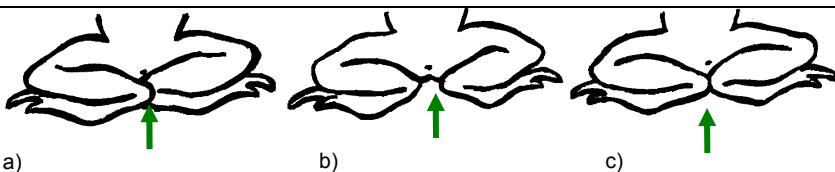
1.att. a) locītavas pārklājas; b) locītavas nesaskaras; c) locītavas saskaras (Pēc Terentyev, Chernov 1949).
